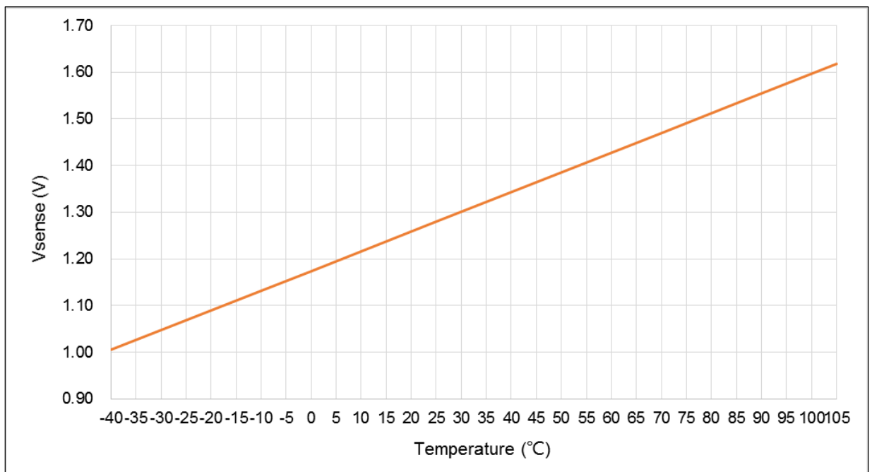
图 1. AT32F415 V_{TS} 对温度理想曲线图
