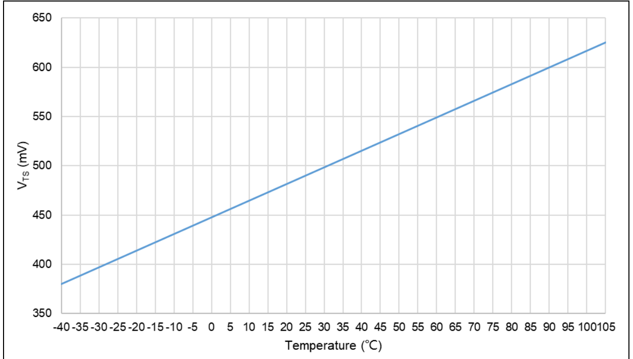
图 2. AT32F490 V_{TS} 对温度理想曲线图
